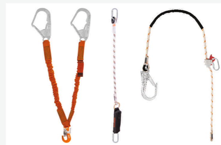
ZACHYCOVACÍ A VYMEZOVACÍ PRACOVNÍ LANA
